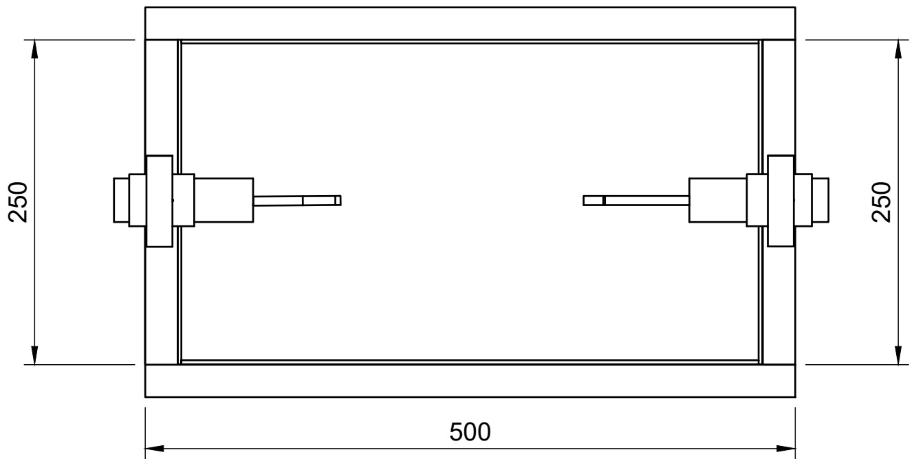
Draufsicht
